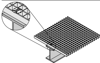
Fixation de caillebotis carré
