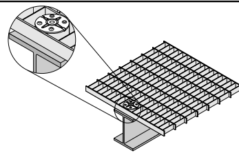
Sicherung rechteckiger Gitterroste
